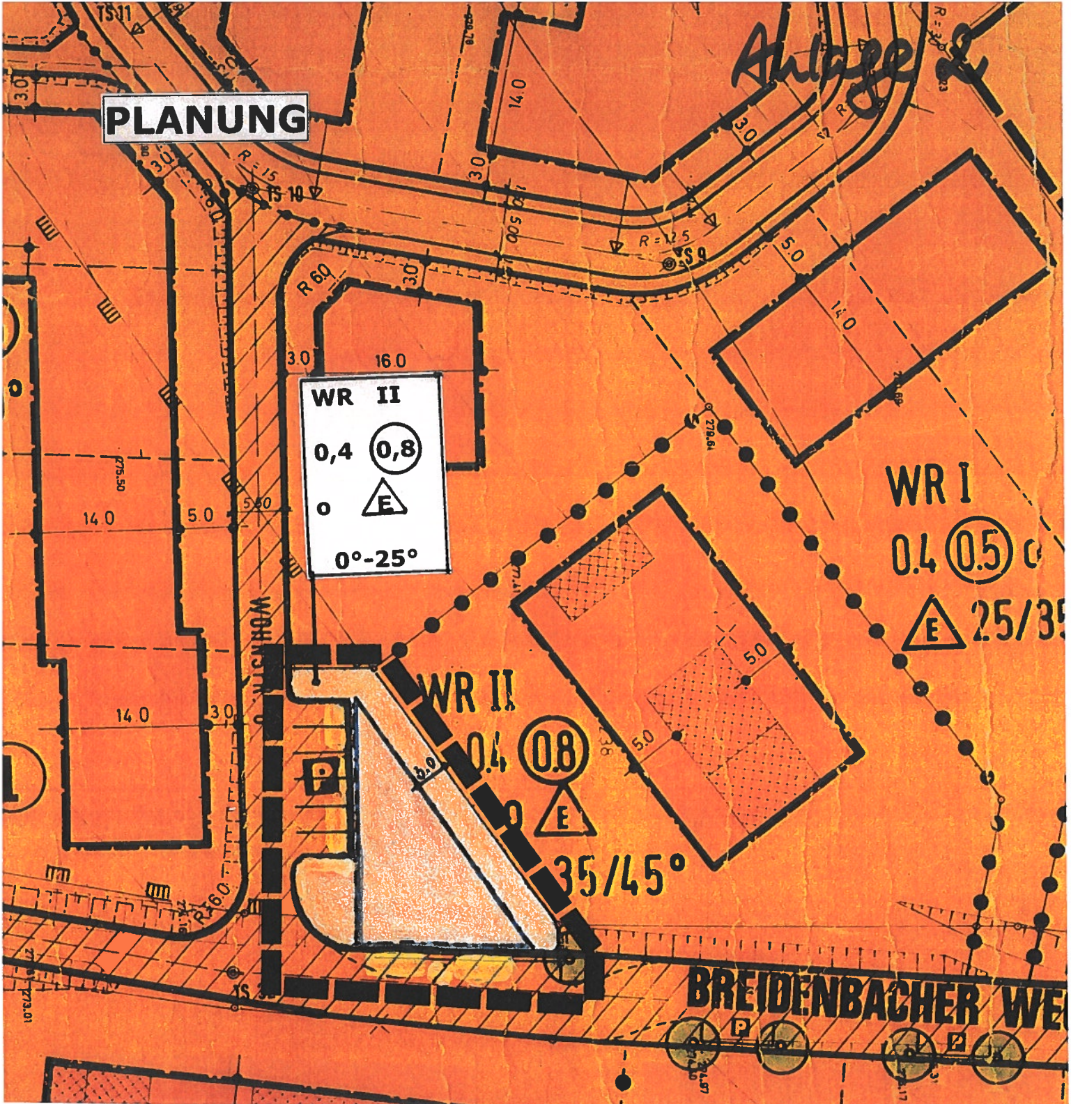
1. Änderung des Bebauungsplanes Nr. 30 – Nümbrecht/West – gem. § 13 a BauGB M. 1 : 500
